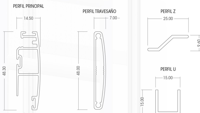
DIMENSIONES DE LA MOSQUITERA
