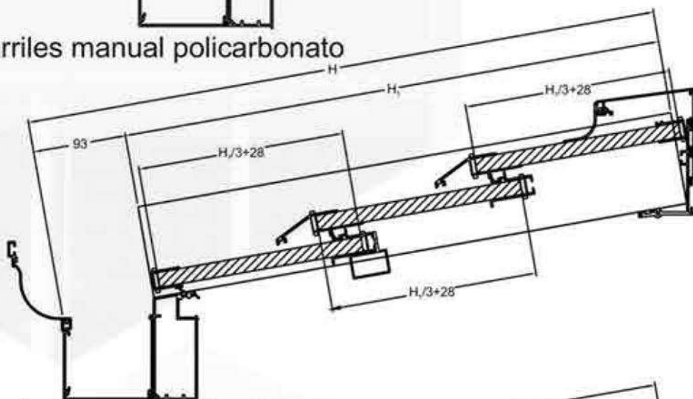
4 Carriles manual policarbonato
