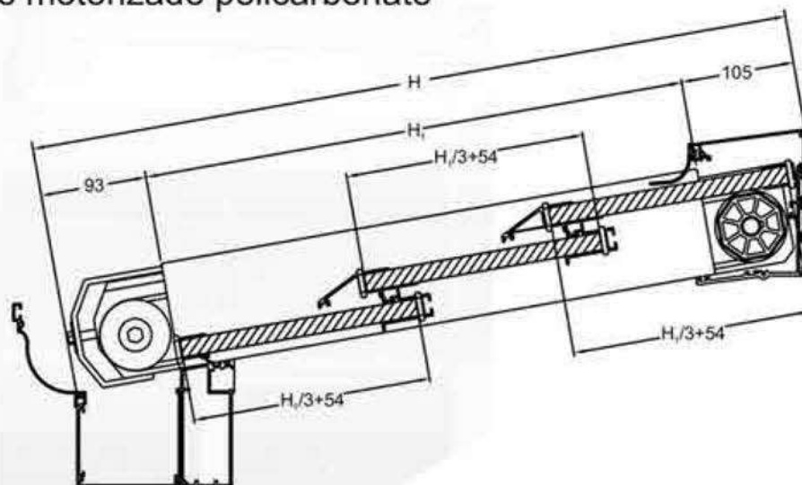
3 Carriles motorizado policarbonato
